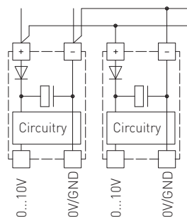
Schéma de raccordement en parallèle
