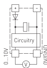
Schéma de raccordement individuel
